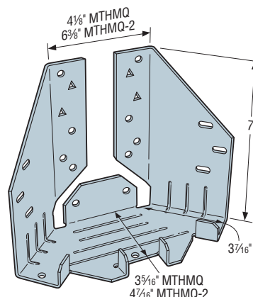
MTHMQ-SDS3 (MTHMQ-2-SDS3 similar)
